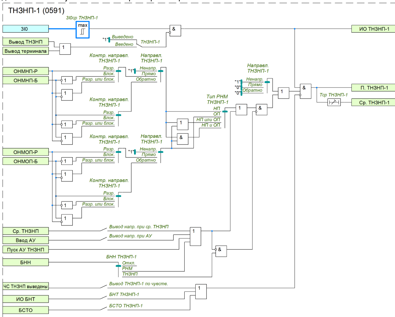
Рисунок 1.19 – Функциональная схема ступени ТНЗНП-1
