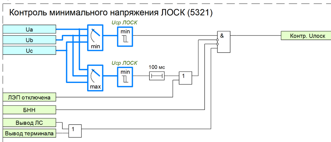
Рисунок 1.38 – Функциональная схема контроля минимального напряжения ЛОСК
